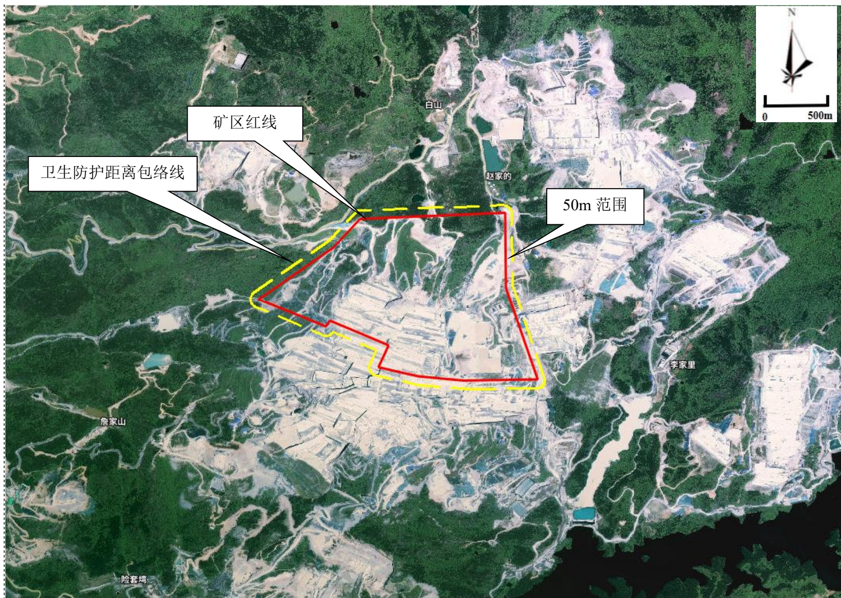
附图 6 项目卫生防护距离包络线图
