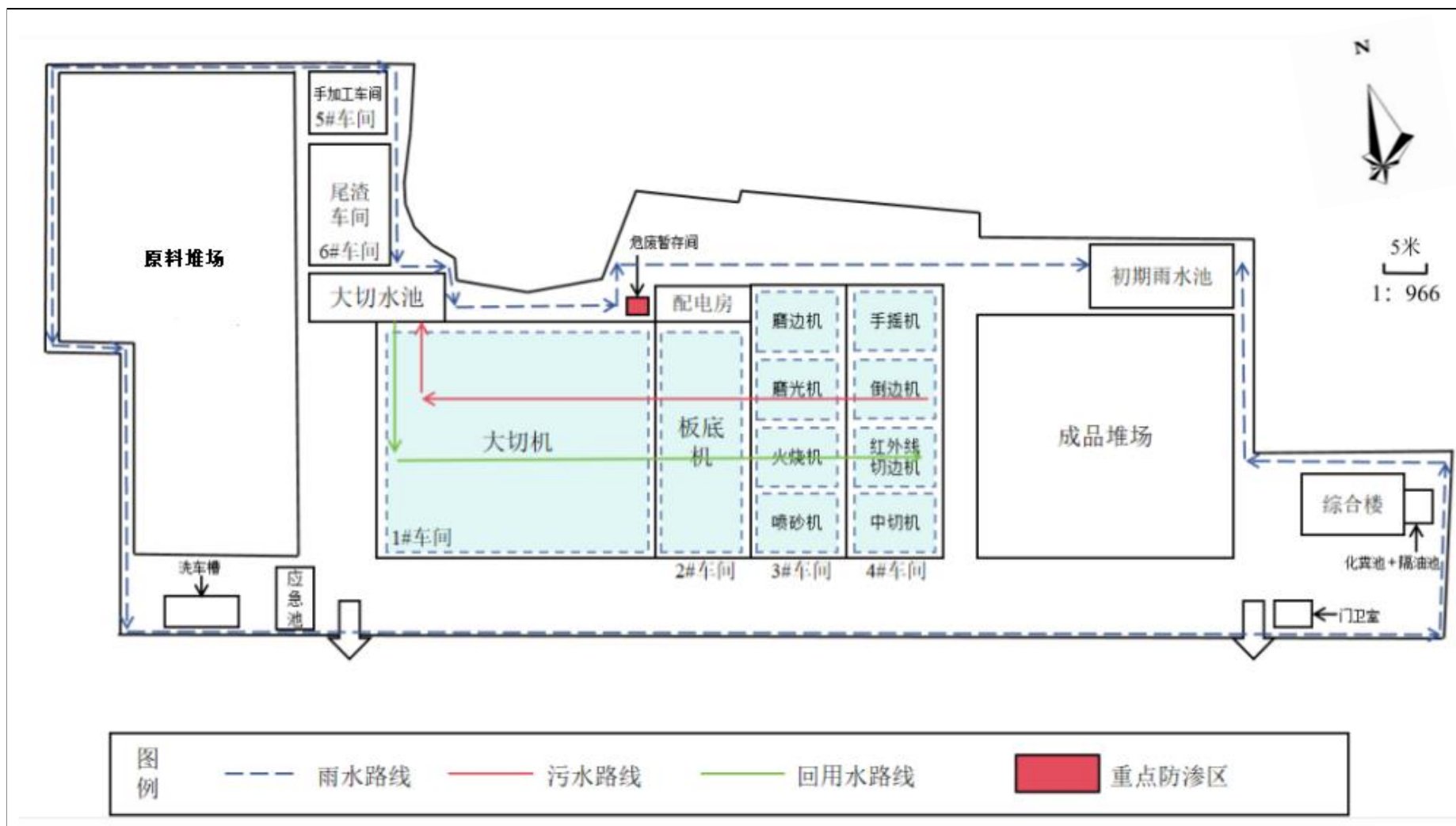
附图3 项目平面布置图及雨污管网图
